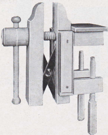
N° 95 ÉTAU A 2 PRESSES, VIS BOIS ET CROISILLONS FER FORGÉ
